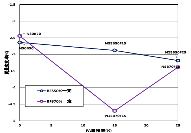
図-2 FA置換による質量変化
