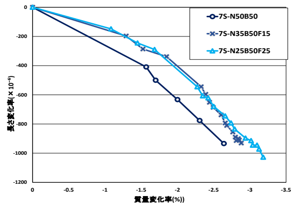
図-3 質量変化-乾燥収縮(BFS50%一定)
