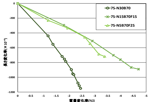
図-4 質量変化-乾燥収縮(BFS70%一定)
