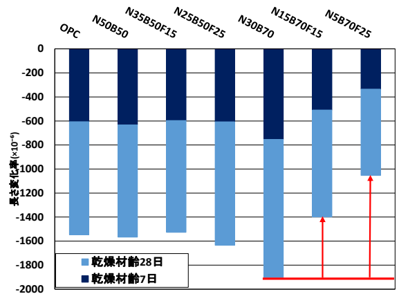
図-1 乾燥収縮量(乾燥期間 28 日)
